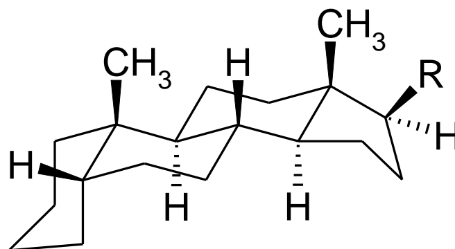
cis-trans-trans cis-trans-trans
