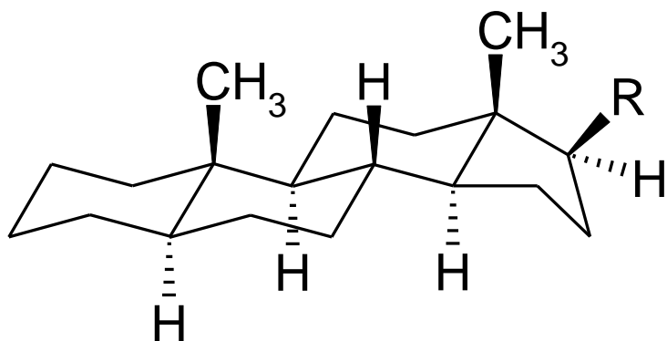
trans-trans-trans trans-trans-trans
