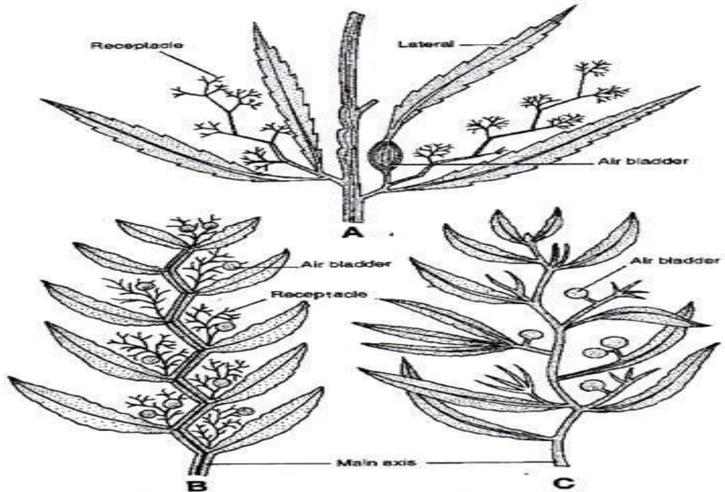
Fig. 2. (A–C). Sargassum . External features. (A) S. longifolium ; (B) S. enerve , (C) S. tenerrimum .
